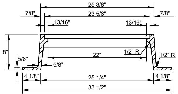
SECTION "A"- "A" MANHOLE FRAME
